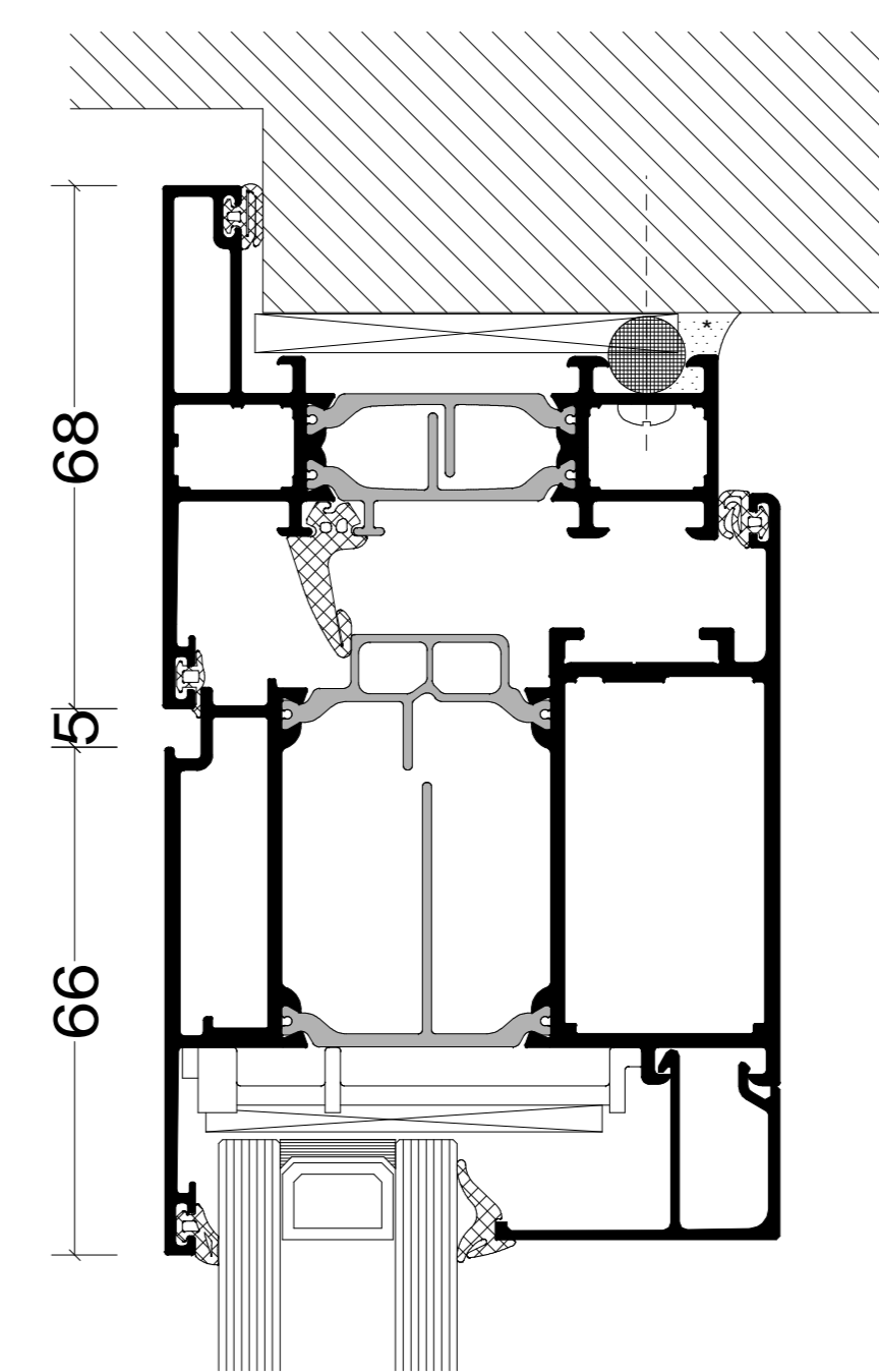
AANSLUITING BOVEN
