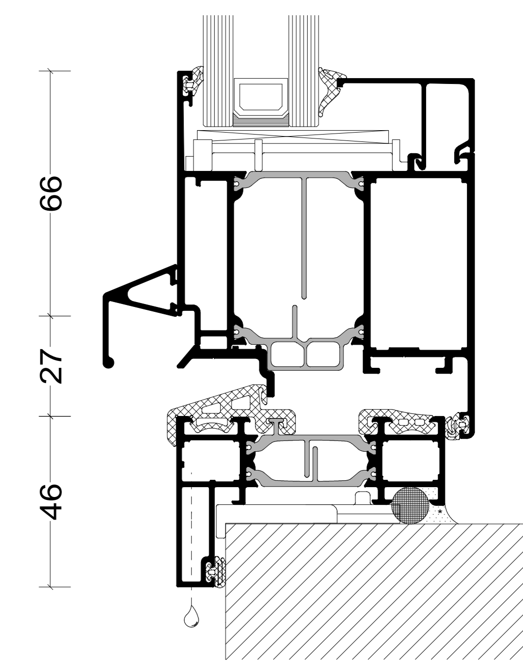
AANSLUITING ONDER
